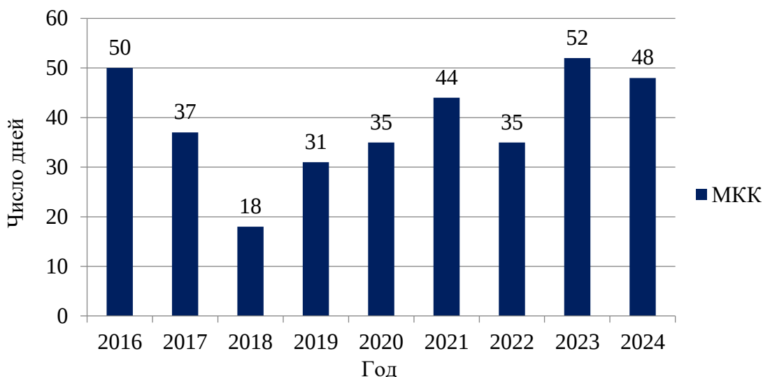
Рисунок 2 – Число дней с мезомасштабными явлениями за теплый период 2016-2024 гг. по данным спутника Meteosat-8 (составлено автором)
