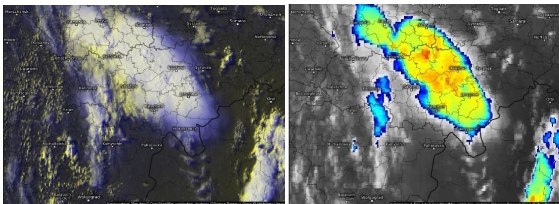
Рисунок 1 – Внешний вид МКК + скопления кучево-дождевых облаков со спутника Meteosat-8, 29 июня 2021 г., время пролета 15:30 UTC [3]
