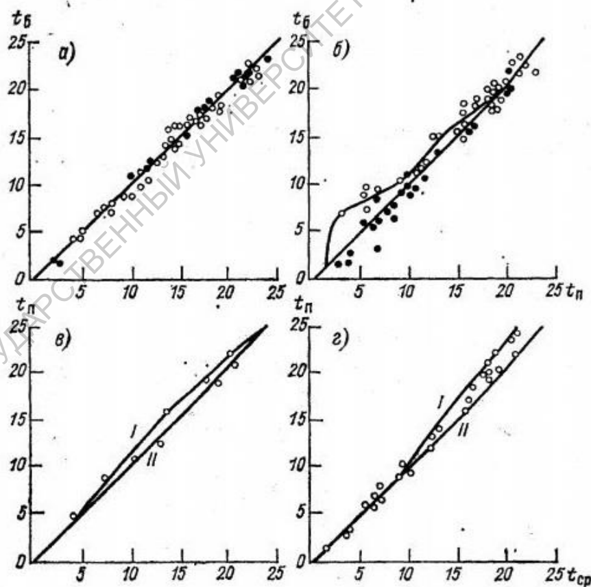
Рис. 3.3. Зависимости температуры поверхности воды в открытой части ( t_{\text{п}} ) и на гидрологических постах ( t_{\text{б}} ) и температуры водной массы ( t_{\text{ср}} ) и температуры поверхности воды ( t_{\text{п}} ) для верхневолжских водохранилищ.
