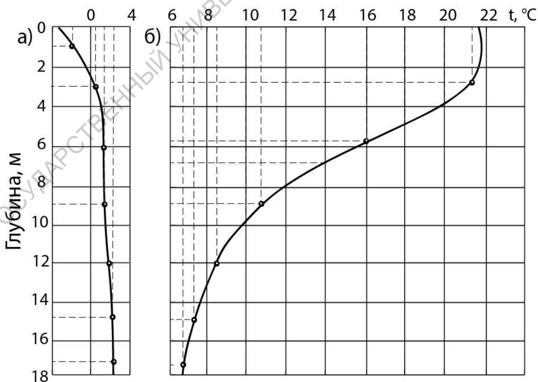
Рис.1. Графики распределения температуры на рейдовой вертикали оз. Светес – х. Спидолес 10/V (а) и 20/VI (б) 1964 г.
