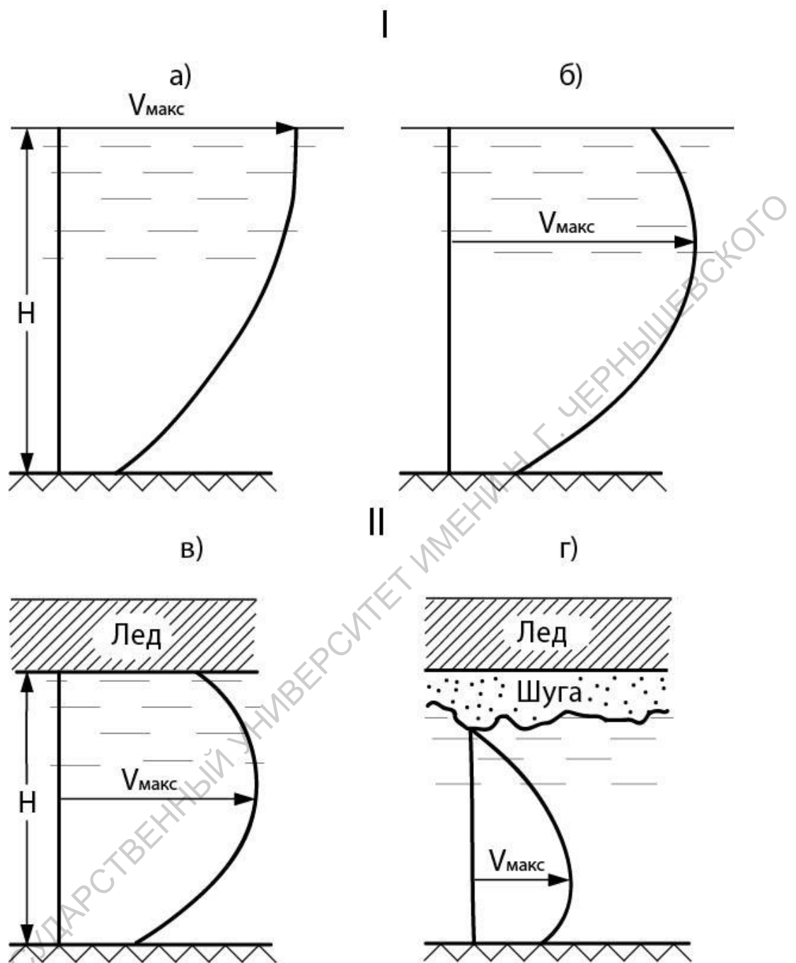
Рис. 1.2 Распределение скоростей течения по вертикали.
